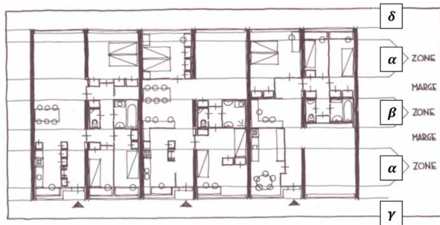
FIGUUR 2.5 Zones en marges (Bron: Boekholt, Denken in Varianten, 1974, pag. 42)
