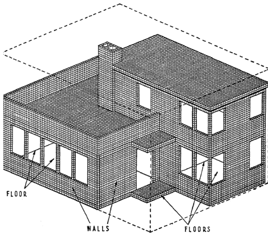
FIGUUR 2.6 Moduulgroepen van het casco (Bron: Bemis, 1933, pag. 73)
